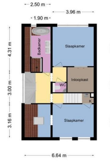
Verloren van Themaatlaan 13, Velsen - Zuid 1e verdieping
